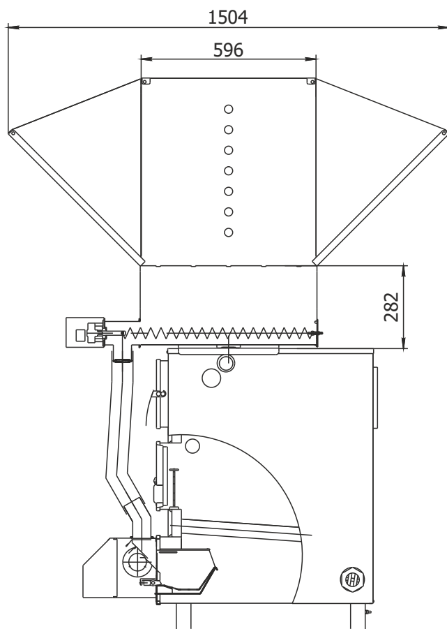
Рис. 4. Установка пеллетной горелки на котел.
