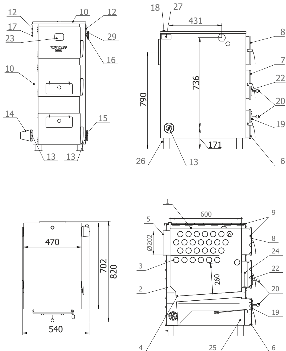
Рис. 3. Конструкция котла КУPPER ПРО 42
